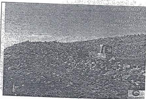
Compactação do lixo. — Aterro Sanitário de Ituiutaba-MG.
