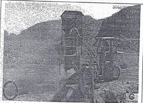
Material sendo triturado. — Aterro Sanitário de Ituiutaba-MG.
