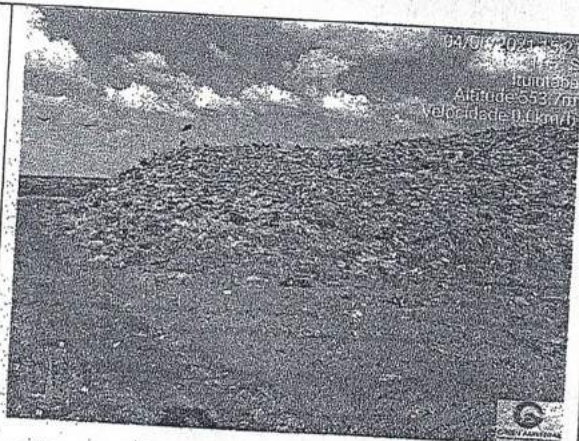
Ponta da célula de lixo domiciliar. — Aterro Sanitário de Ituiutaba-MG.
