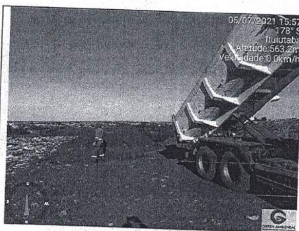
Realização da cobertura da lateral do lixo. — Aterro Sanitário de Ituiutaba-MG.
