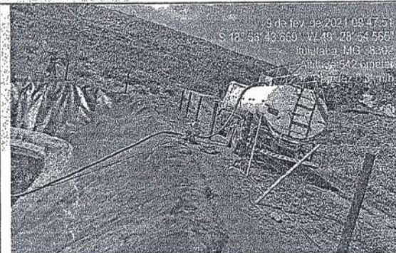
Retirada Chorume para ERPAI. — Aterro Sanitário de Ituiutaba-MG.
