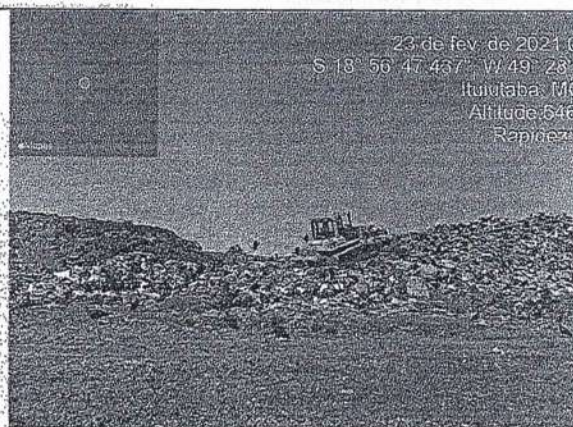
Compactação do lixo domiciliar. — Aterro Sanitário de Ituiutaba-MG.
