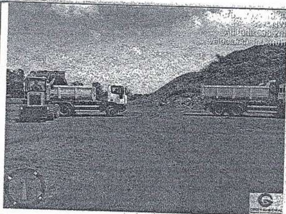
Retirada do RCC.— Aterro Sanitário de Ituiutaba-MG.
