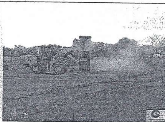
Material sendo colocado para realizar a trituração. – Aterro Sanitário de Ituiutaba-MG.
