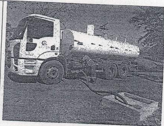
Descarte do chorume na ERPAL. — Aterro Sanitário de Ituiutaba-MG.
