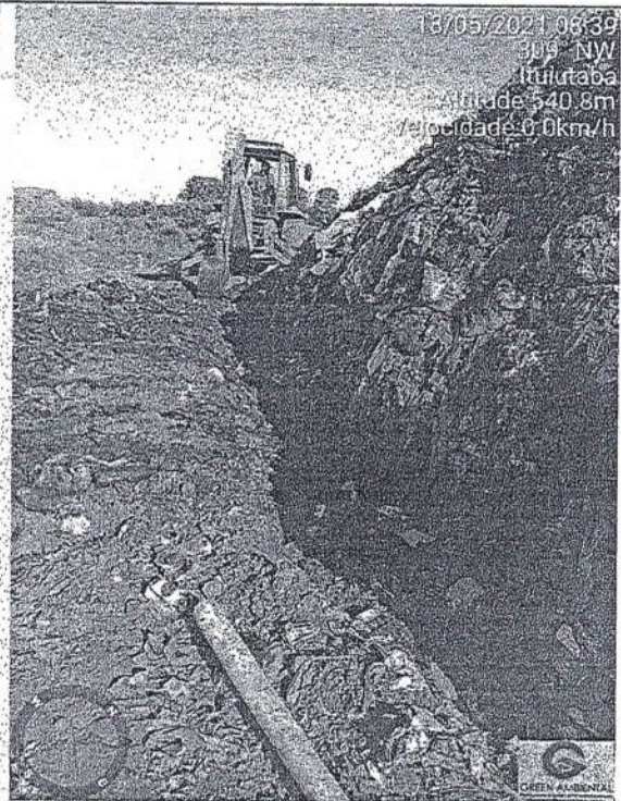
Drenagem no pé do talude. — Aterro Sanitário de Ituiutaba-MG.
