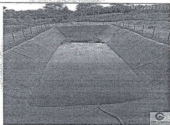
Lagoa com nível controlado – Aterro Sanitário de Ituiutaba-MG.
