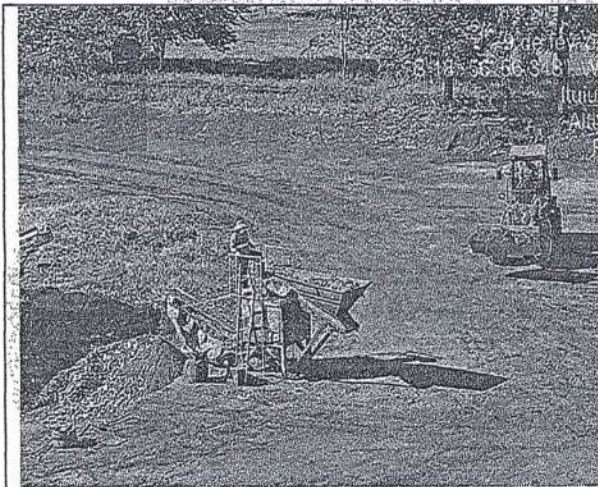
Britagem para RCC.. — Aterro Sanitário de Ituiutaba-MG.
