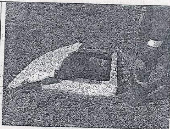
Limpeza caixa de drenagem do chorume. – Aterro Sanitário de Ituiutaba-MG.
