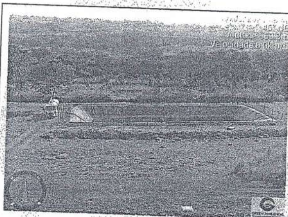
Realizando a retirada do chorume. — Aterro Sanitário de Ituiutaba-MG.
