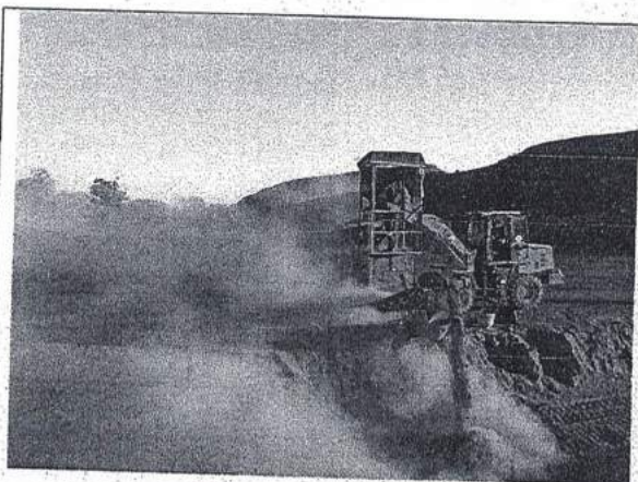
Trituração do entulho. – Aterro Sanitário de Ituiutaba-MG.
