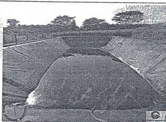
Lagoa de Chorume em seu nível mínimo. – Aterro Sanitário de Ituiutaba-MG.
