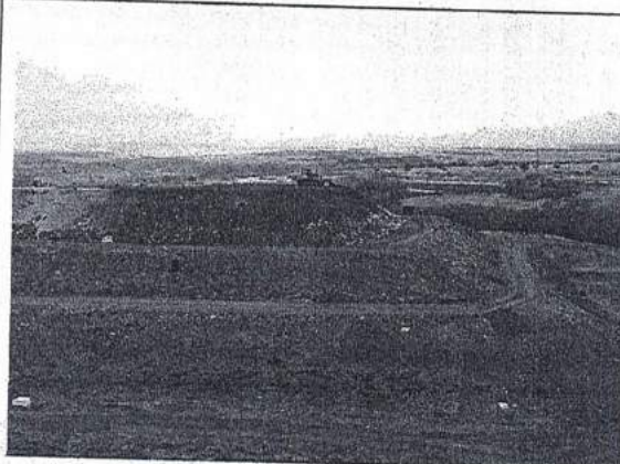
Cobertura completa da célula de lixo. – Aterro Sanitário de Ituiutaba-MG.
