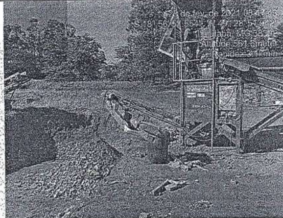
Britagem do Entulho. — Aterro Sanitário de Ituiutaba-MG.
