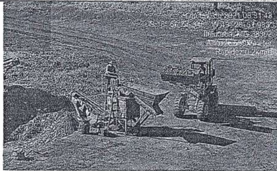
Britagem para RCC. — Aterro Sanitário de Ituiutaba-MG.
