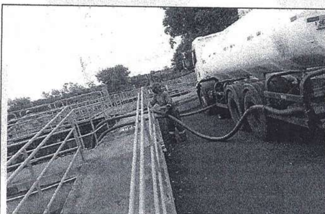
Descarte de chorume. – Aterro Sanitário de Ituiutaba-MG.
