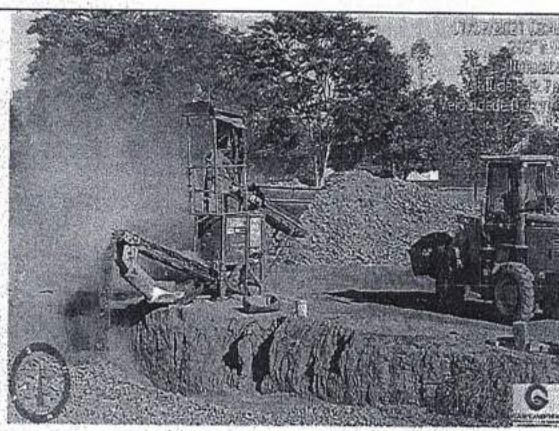
Realizando a trituração. – Aterro Sanitário de Ituiutaba-MG.
