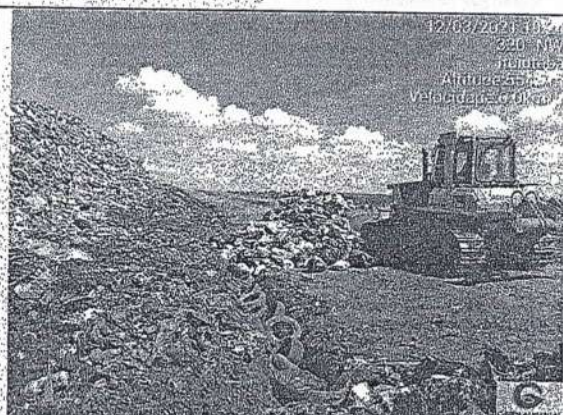
Espalhamento de lixo em cima da drenagem realizada. — Aterro Sanitário de Ituiutaba-MG.
