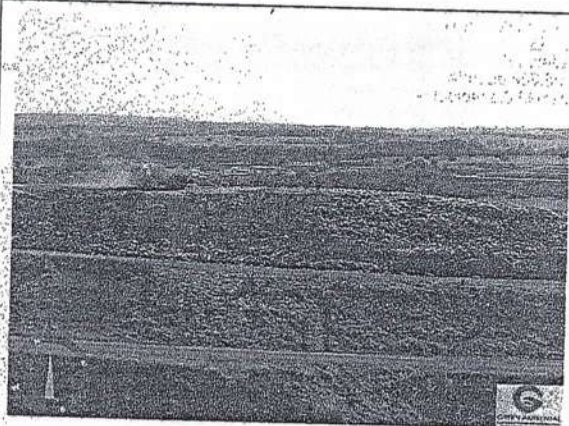
Realizando a cobertura com terra na lateral da célula. – Aterro Sanitário de Ituiutaba-MG.
