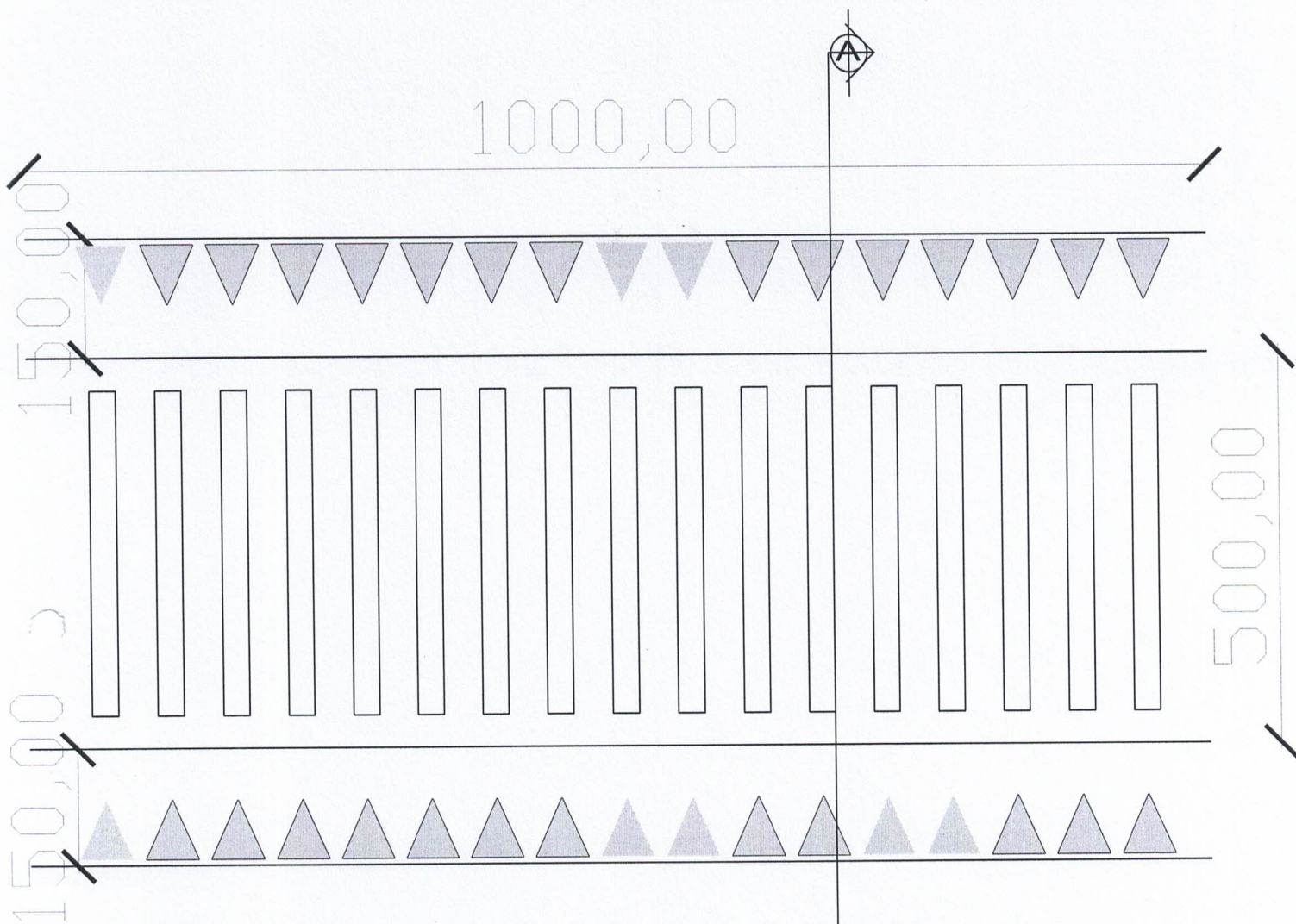
PLANTA BAIXA MEDIDAS EM CM SEM ESCALA
